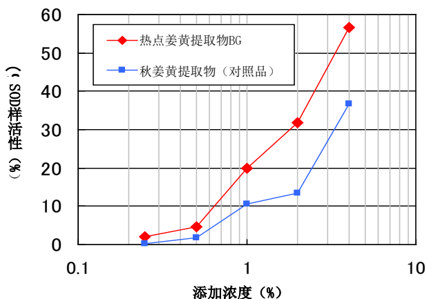
①SOD活性
