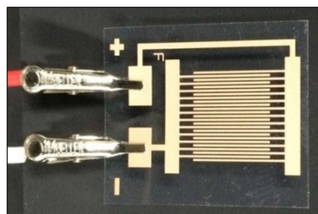
（当社銅ペースト：L/S: 316 μm/316 μm）
