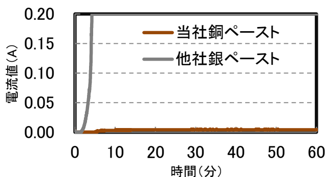
ウォータードロップ試験結果（印加電圧：2 V）
