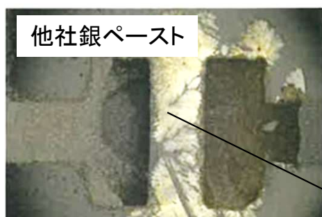
ウォータードロップ試験（印加電圧：2 V） 電極間距離：316 (μm)
