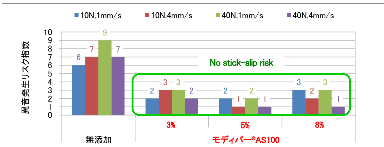
図4. スティック・スリップ試験による異音防止性評価
