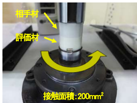
図 3. 滑り摩耗試験機
