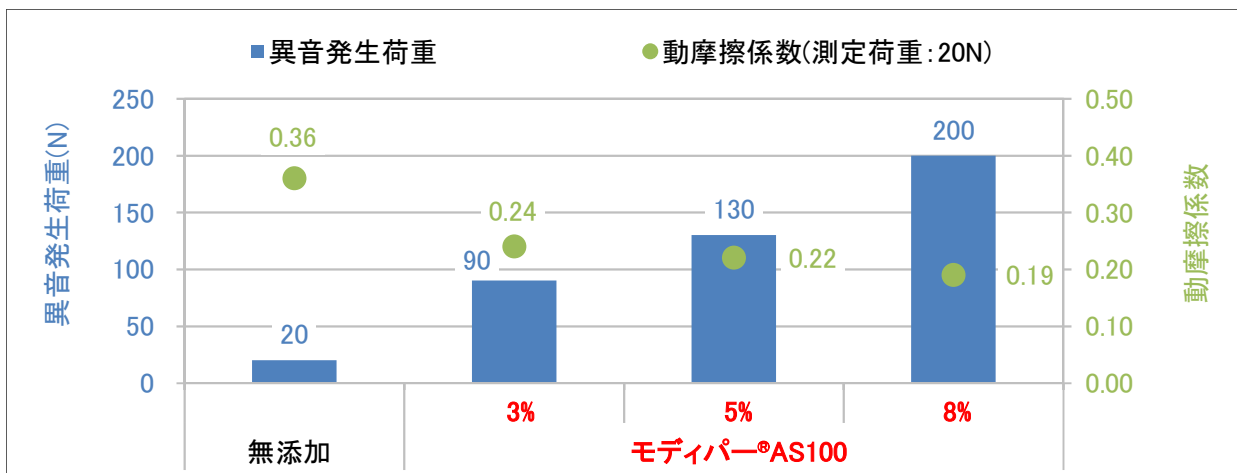
図5. リング・オン・リング試験による異音防止性評価
